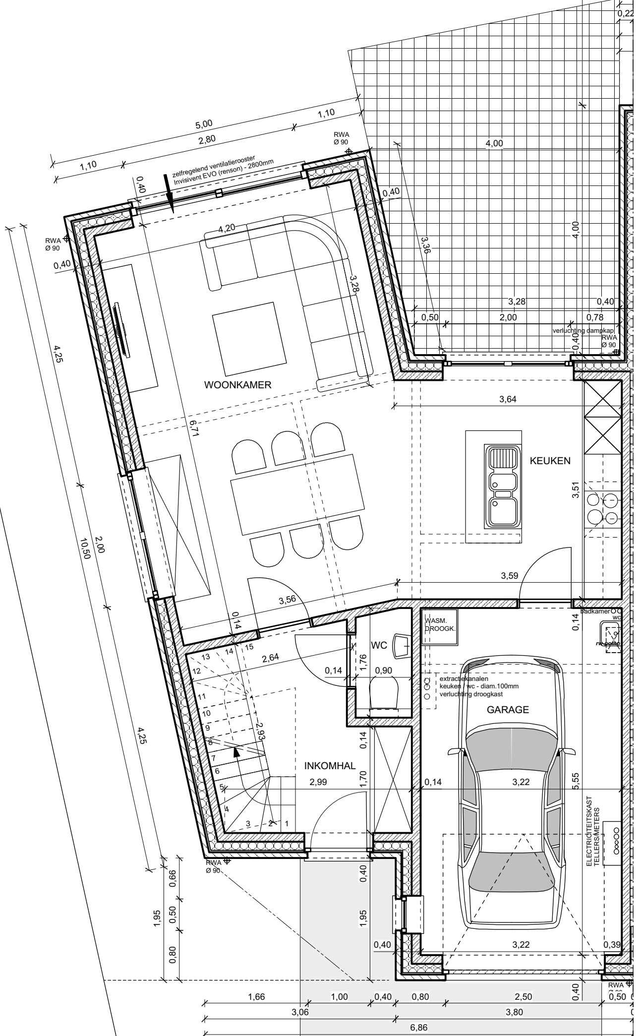
GRONDPLAN WONING LOT 1 NETTO VLOEROPPERVLAKTE GELIJKVLOERS = 70,00m 2
