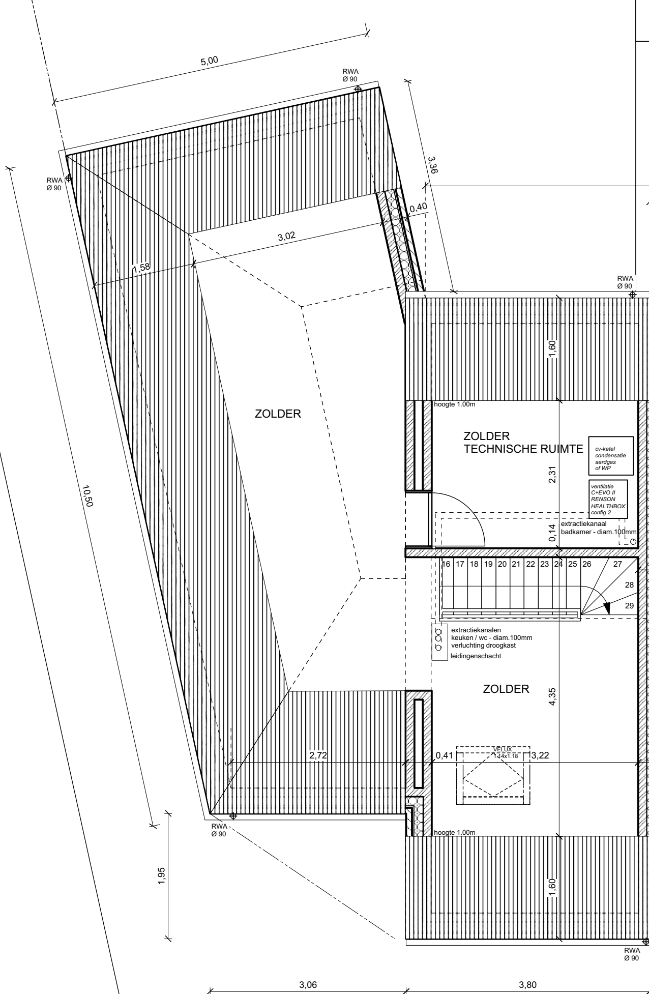
ZOLDERPLAN WONING LOT 1 NETTO VLOEROPPERVLAKTE ZOLDER = 43,00m 2
