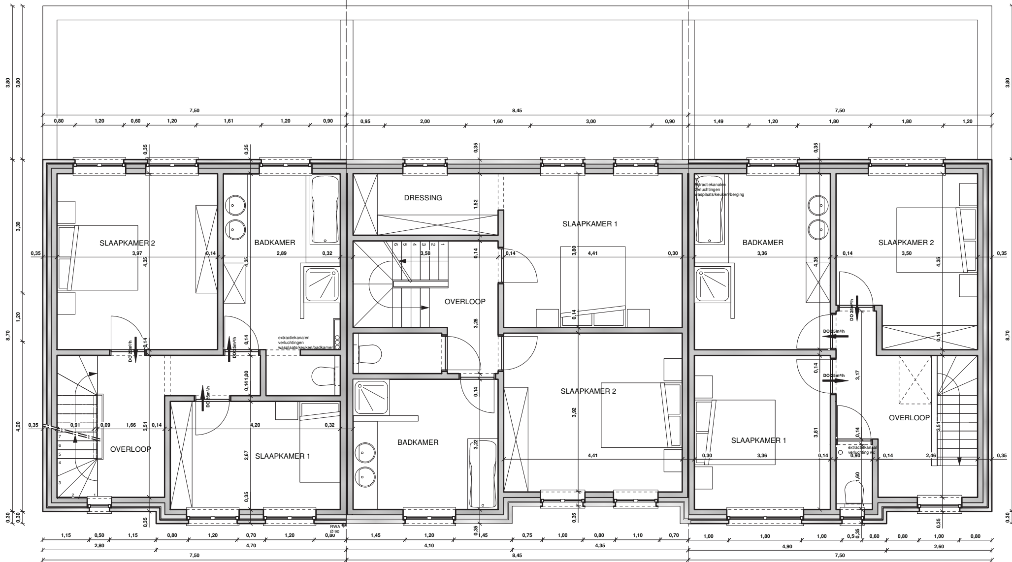
VERDIEPINGSPLAN schaal 1/65
