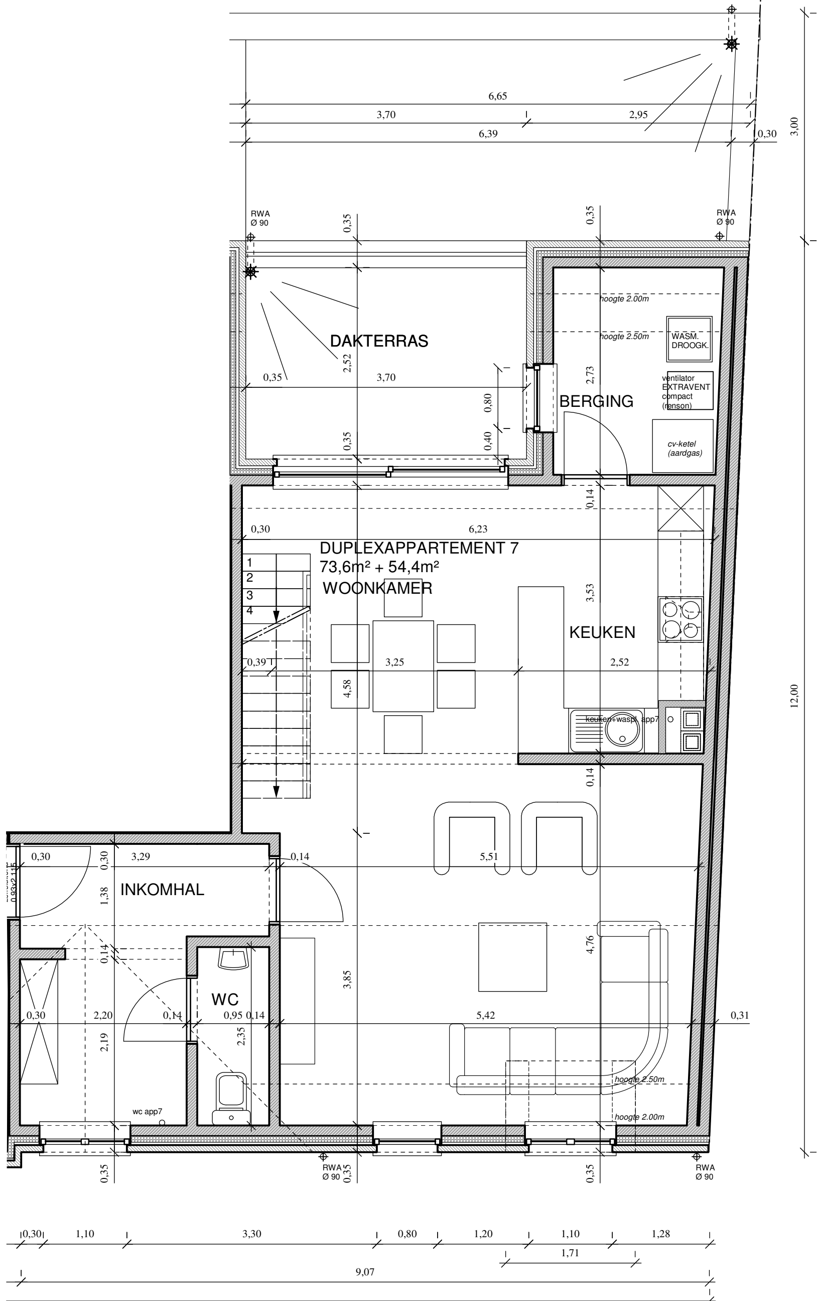
GRONDPLAN DUPLEXAPPARTEMENT 7
