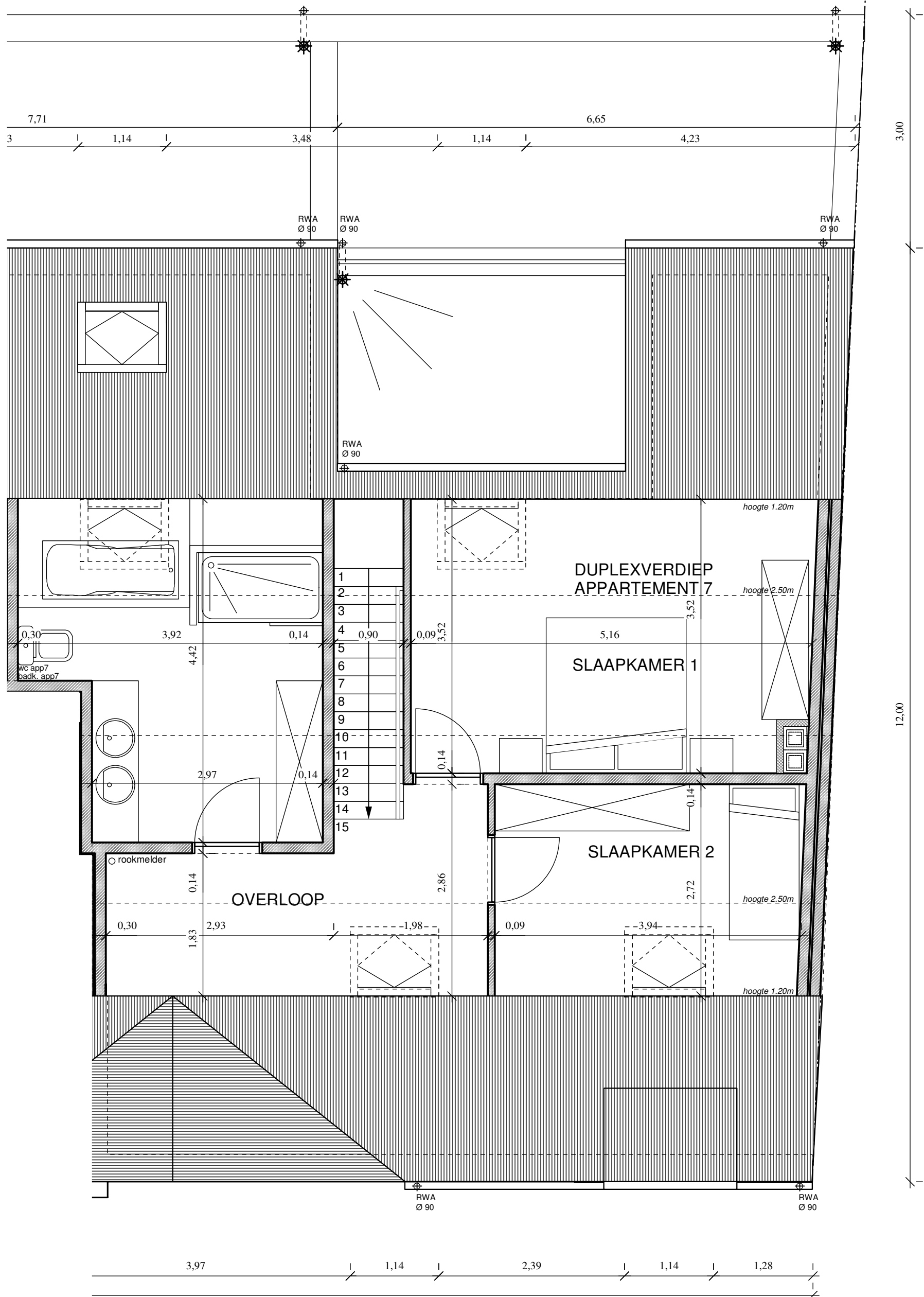
VERDIEPINGSPLAN DUPLEXAPPARTEMENT 7
